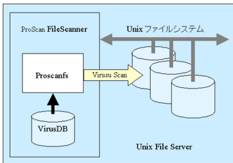
図1 Filescannerの内部アーキテクチャ
